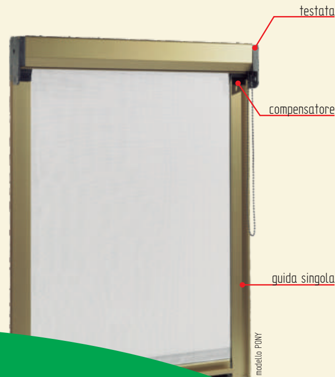
Scomparsa superiore con catenella frizionata
